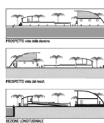
SEZIONE LONGITUDINALE
